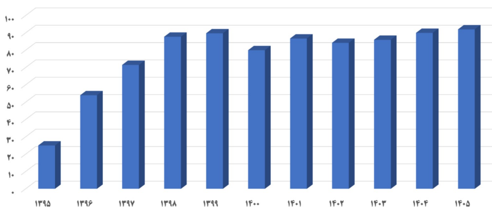
نمودار درصد تشابه واژگان مورد استفاده در آزمون‌های زبان دکتری نسبت به دوره‌های گذشته
